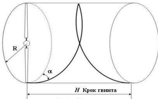
Рис. 2.48. Крок гвинта
