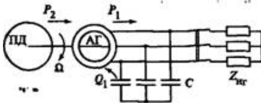
Рис. 2.9. Схема включення асинхронного генератора при роботі з самозбудженням: АГ – асинхронний генератор; ПД – приводний двигун; C – конденсатори; Z нр – опір навантаження; P 1 та P 2 – потужності; Q 1 – заряд
