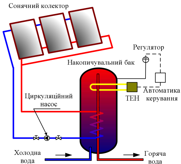
Рис. 3.17. Схема підключення сонячних колекторів до системи ГВП: a – до двоконтурного котла; б – до електричної системи підігріву
