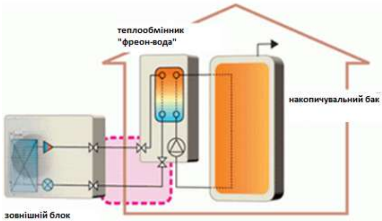
Рис. 4.17. Схема приєднання додаткового обладнання
