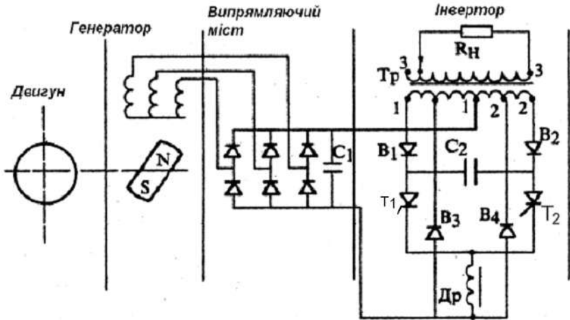
Рис. 2.21. Принципова схема синхронного генератора з постійними магнітами та інвертором
