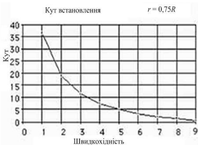
Рис. 2.38. Залежність кута встановлення лопаті від швидкохідності
