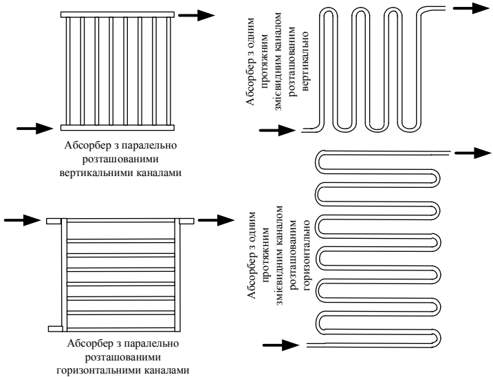
Рис. 3.9. Розташування проточних каналів в абсорбері
