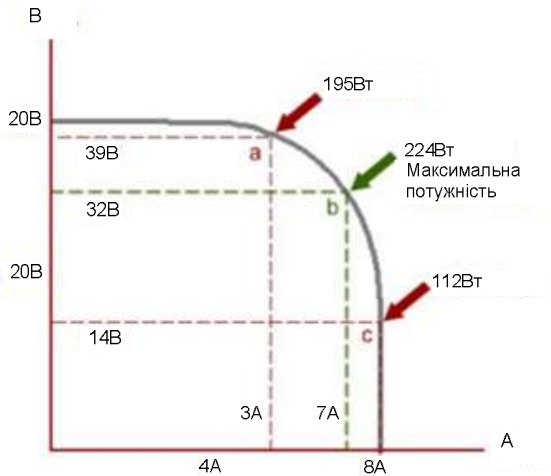
Рис. 3.39. Коригування потужності інвертора
