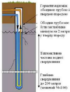
Рис. 4.20. Розміщення колектора
