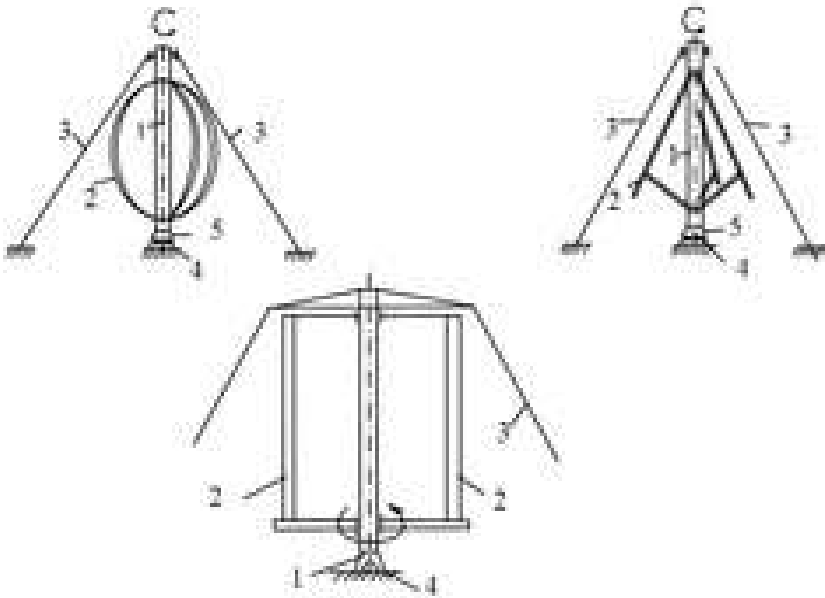
Рис. 2.51. Вітроенергетичні установки (Дар'є) з вертикальним ротором a – \Phi -подібний; б – D -подібний; в – з прямими лопатями. 1 – вежа; 2 – ротор; 3 – розтяжки; 4 – опора (фундамент); 5 – генератор
