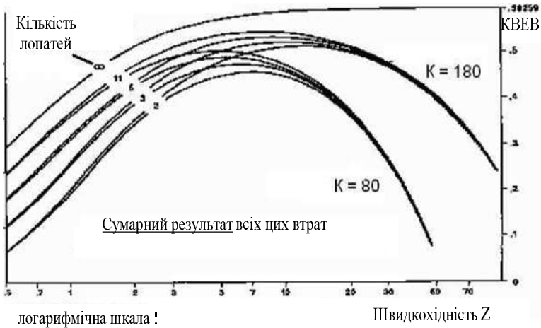
Рис. 2.42. Залежність коефіцієнта використання енергії вітру від швидкості
