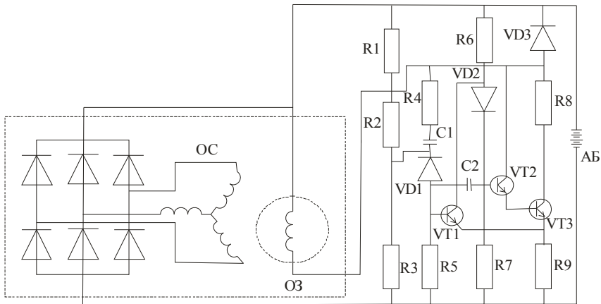
Рис. 2.16. Принципова схема генератора з регулятором напруги: ОС – обмотка статора; ОЗ – обмотка збудження; АБ – акумуляторна батарея; VD1 – стабілітрон
