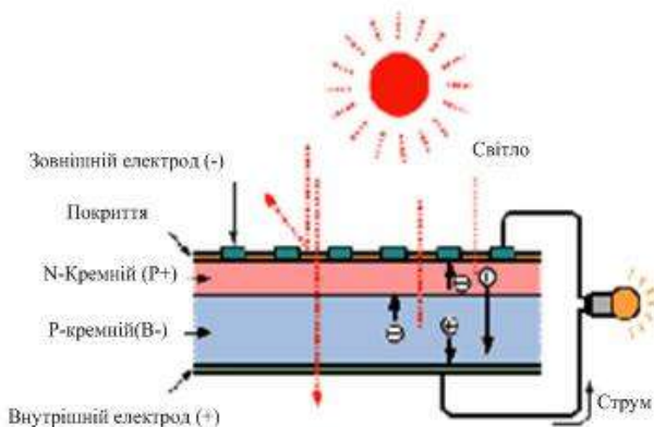
Рис. 3.29. Фотоелемент
