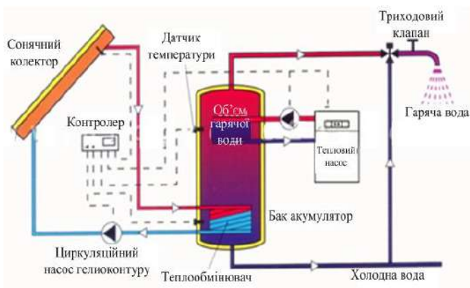
Рис 3.7. Структурна схема системи з використанням сонячного колектора
