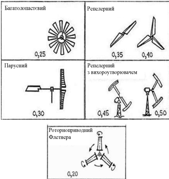
Рис. 2.13. Коефіцієнти використання вітру для горизонтально-осьових ВЕУ
