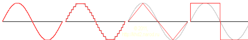
Рис. 3.48. Форми напруги на виході інвертора: синусоїдальна, синусоїдальна модифікована, трикутна, меандр
